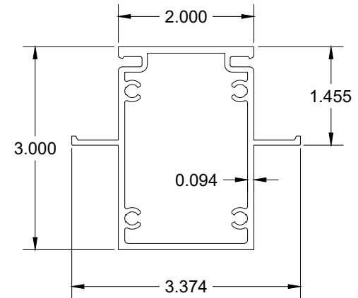
5 DIVIDER STILE
